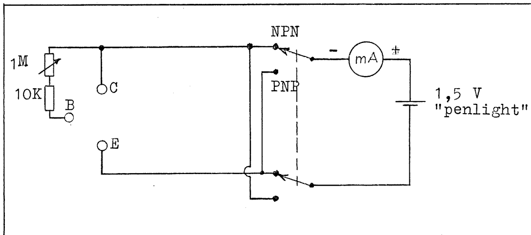
Fig 6 transistorprovare
