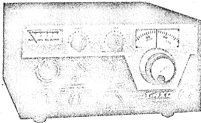
Drake T4XC, amerikansk sändare. 200 W. Täcker alla amatörband upp till 10-metersbandet. (Elfa Radio, Stockholm.)
